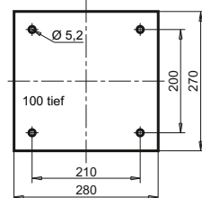
Elektronik - Schaltschrank (Bohrbild)
