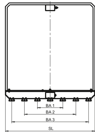
Elektronik - Schaltschrank (Bohrbild)
